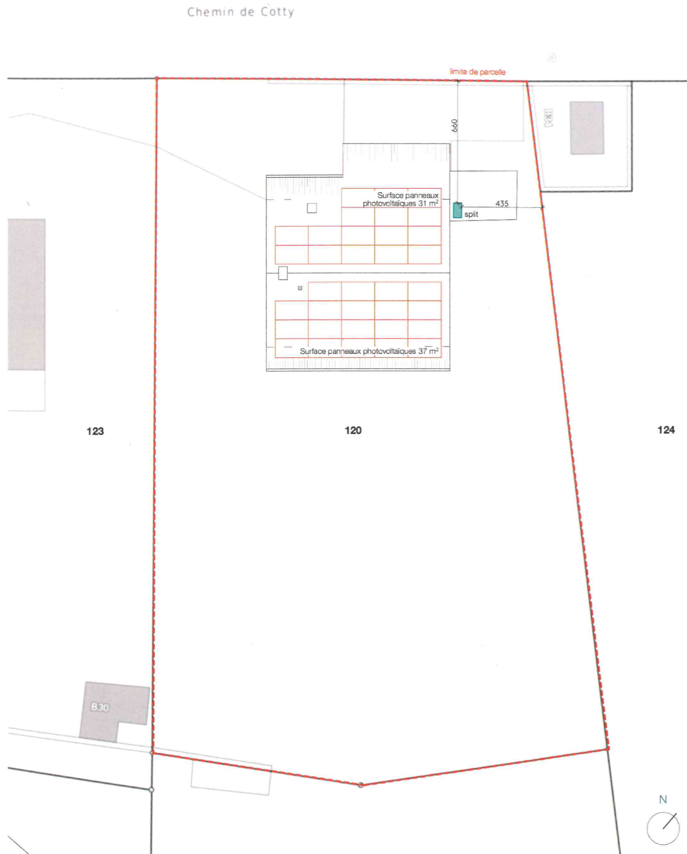
Plan toiture - base géodonnées Etat de Vaud, office fédéral de topographie - www.geo.vd.ch
